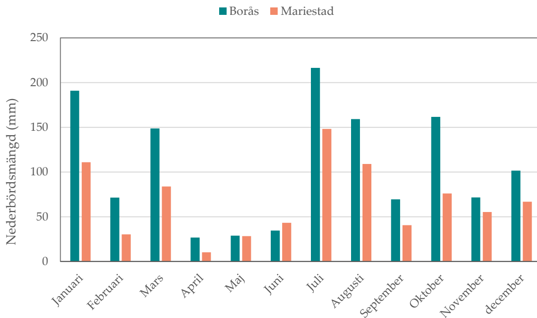
Figur 3 Nederbördsmängd under 2023 vid de närliggande meteorologiska stationerna till Borås och Mariestad.
