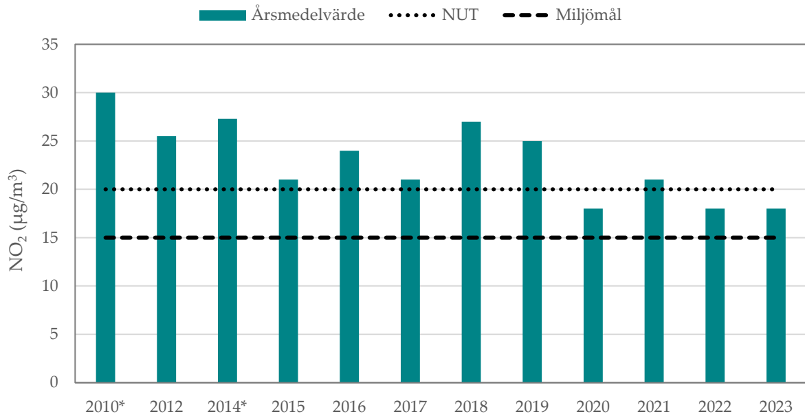
Figur 15 Årsmedelvärden av NO 2 i gaturum i Borås mellan 2010 och 2023. * baserat på mätning av månadsmedelvärden
