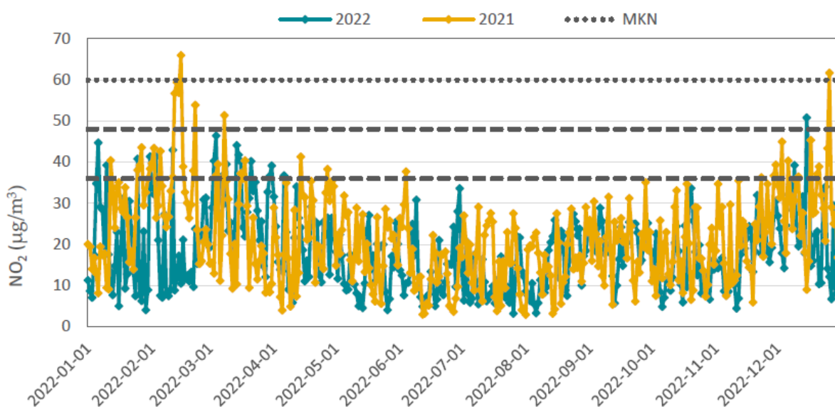
Figur 3. Dygnsmedelvärden av kvävedioxid (µg/m 3 ) i Borås gaturum under 2021 och 2022 samt MKN och utvärderingströsklarna för dygnsmedelvärde.
