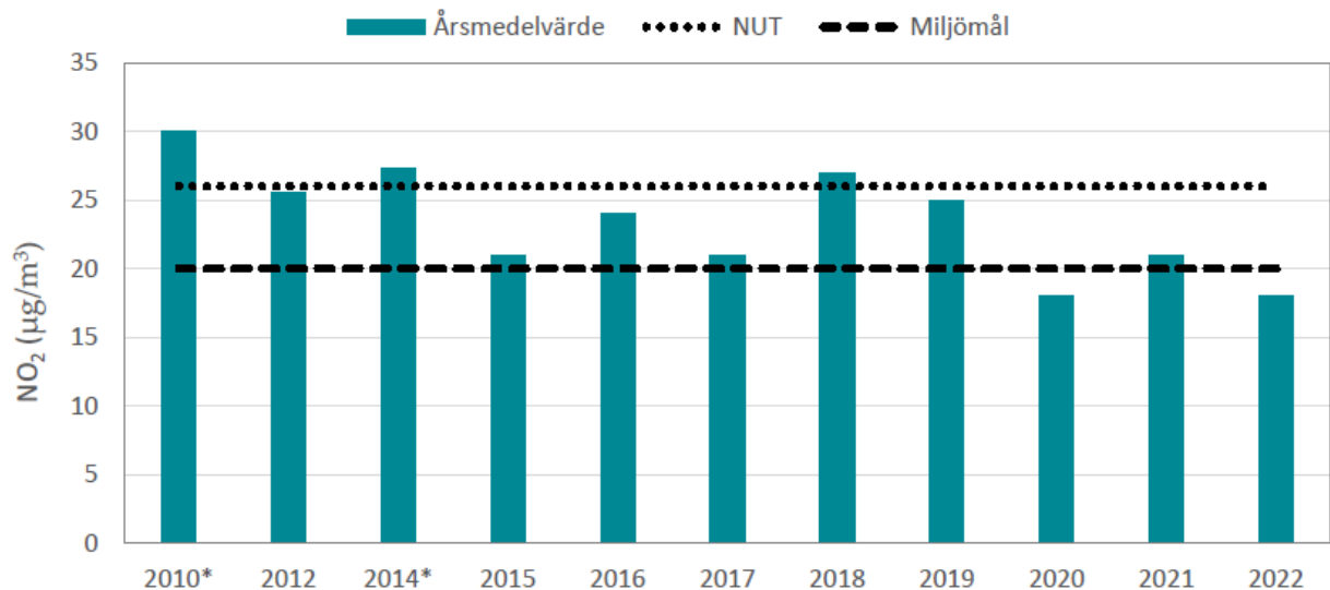
Figur 4. Årsmedelvärden av NO 2 i gaturum i Borås mellan 2010 och 2022.
