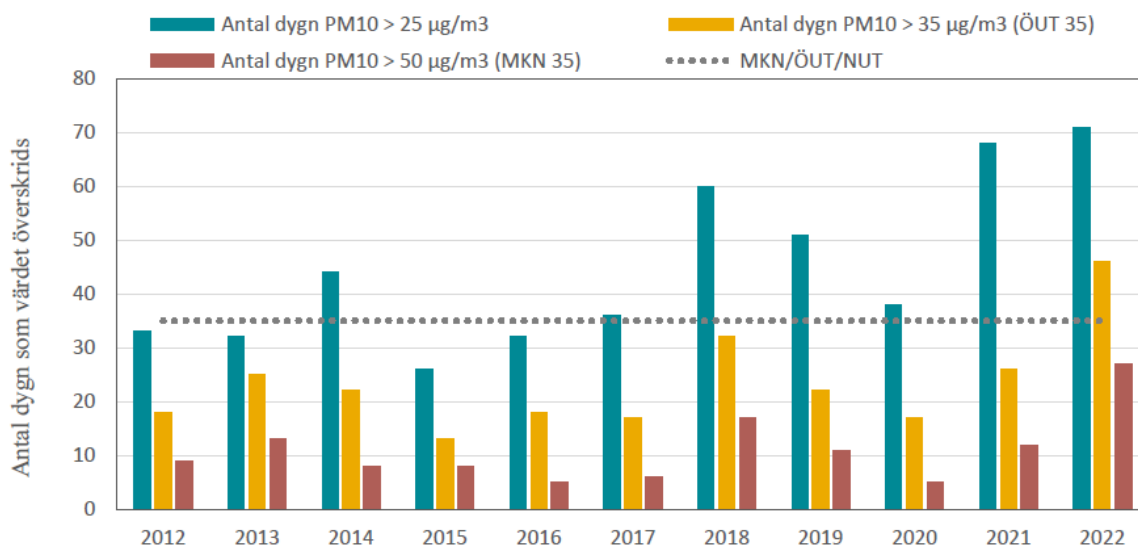
Figur 2. Antal dygns överskridande av MKN, ÖUT och NUT för PM10 som dygnsmedelvärde i gaturum vid Kungsgatan i Borås mellan 2012 och 2022.
