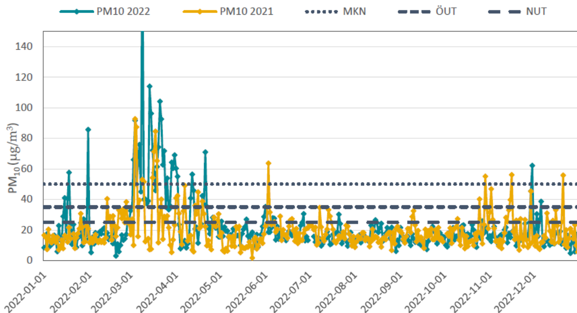
Figur 1. Dygnsmedelvärden av PM 10 ( \mu\text{g}/\text{m}^3 ) i Borås under 2021 och 2022 jämfört med MKN, ÖUT och NUT för PM 10 som dygnsmedelvärde.
